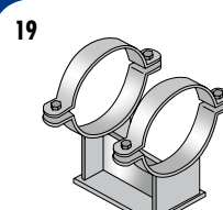
19 Rohrleitlager
