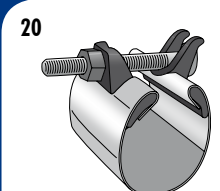
20 Reparaturschellen, Breitbandschellen
